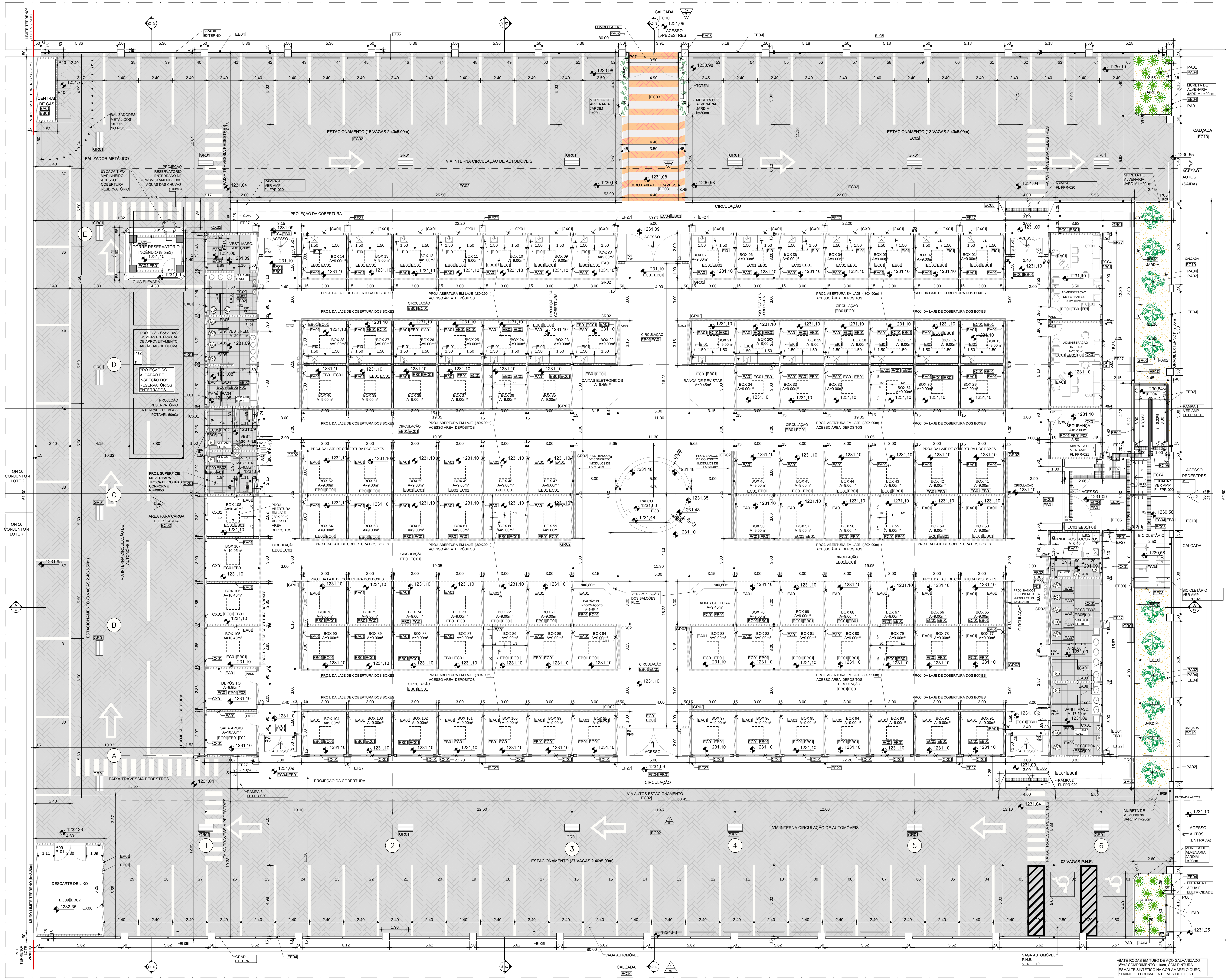
1 PLANTA ESC.: 1:100
