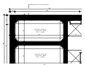
Detalhe - Reservatório de Água ESC. 1:25
